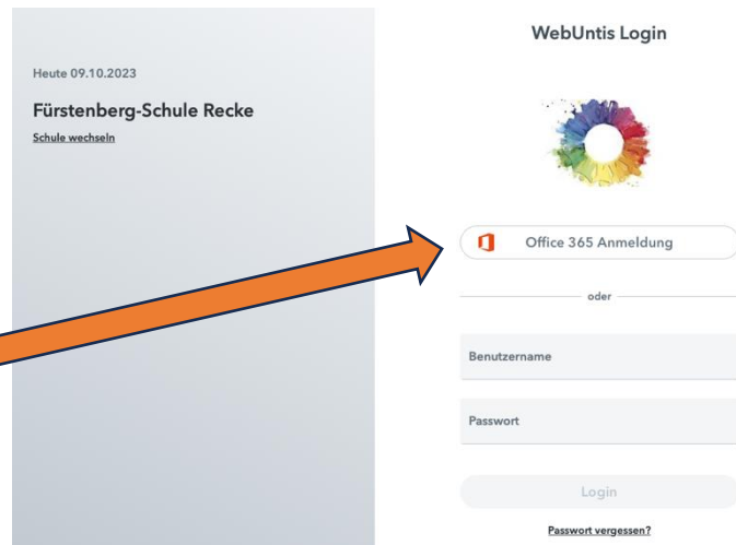
Abbildung 1: Anmeldeseite www.webuntis.com
